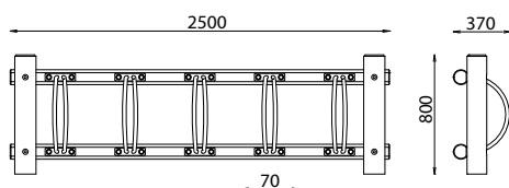
Passage pneus 70mm
